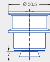
Tri-Clamp-Anschluss
