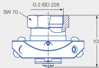
Innengewinde
