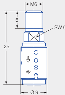
Außengewinde
